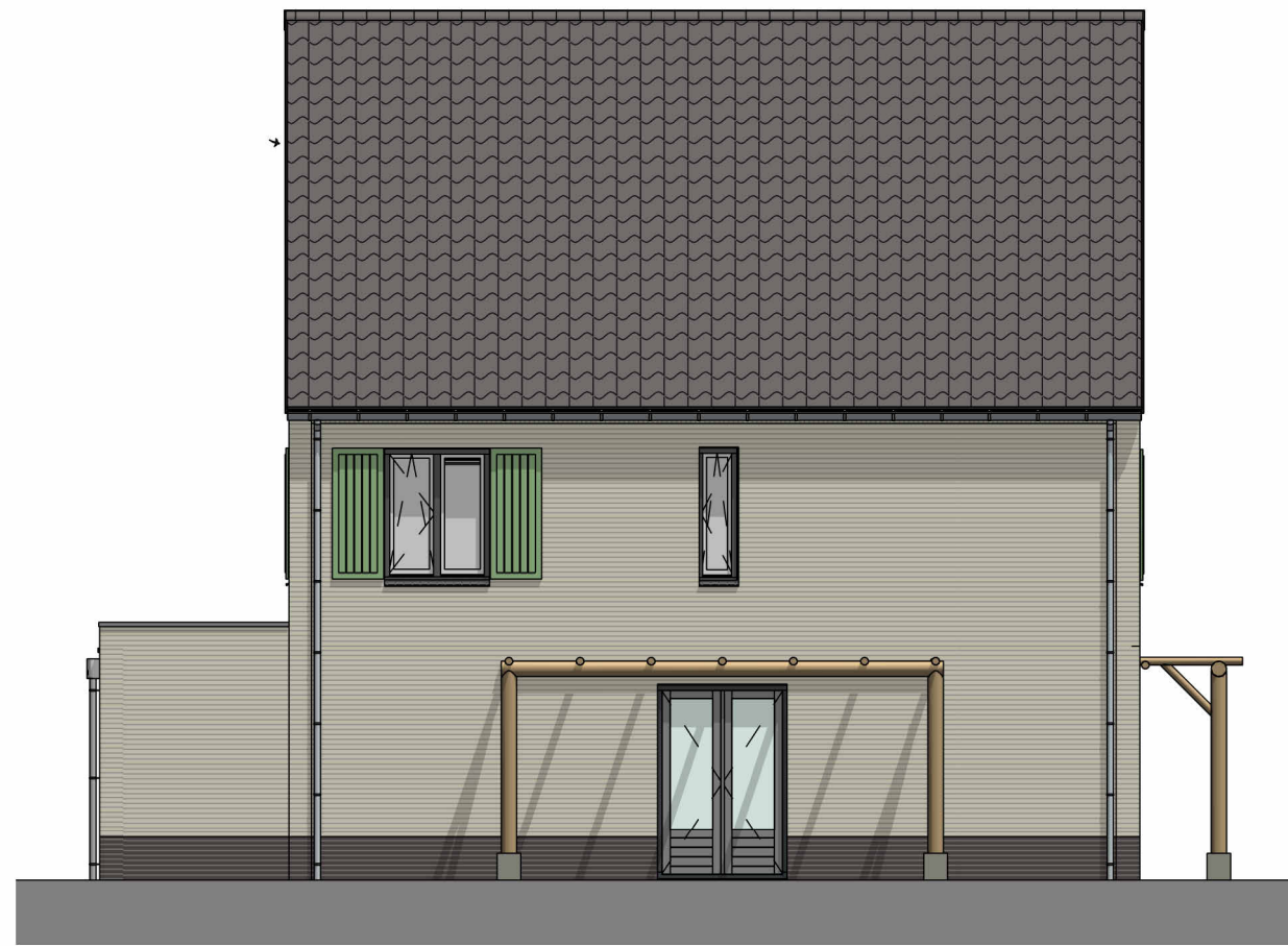
linkergevel met optie uitbreiding achtergevel
